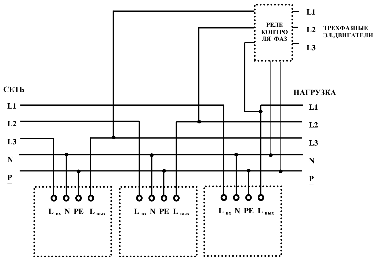
Рис.1 Схема включения однофазных стабилизаторов по схеме “Звезда” для формирования трехфазного стабилизатора. При необходимости устанавливается дополнительный блок реле контроля фаз (опция).
