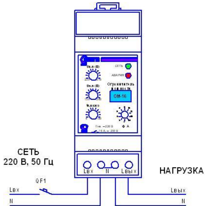
Рис.1. Порядок подключения реле.
