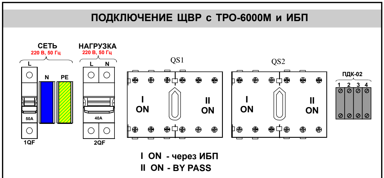
Рис. 1 Схема подключения автоматов и клеммников.
